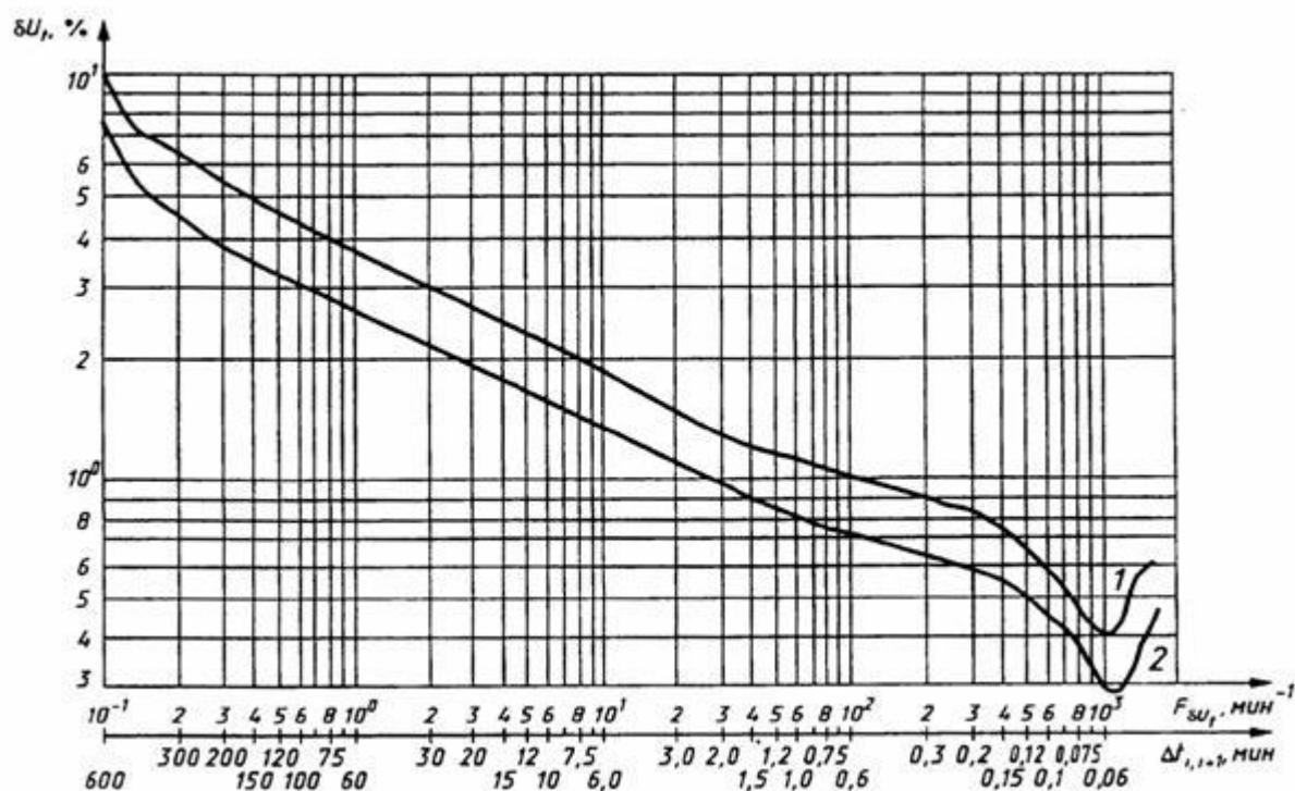
Рисунок 1 - Предельно допустимые размахи изменений напряжения в зависимости от частоты повторения изменений напряжения за минуту для колебаний напряжения, имеющих форму меандра
