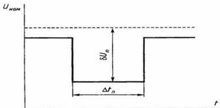
Рисунок Б.2 - Провал напряжения
