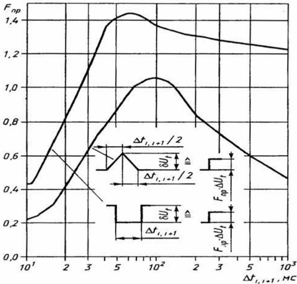
Рисунок В.2 - Коэффициент приведения F_{np} для прямоугольных и треугольных периодических колебаний напряжения
