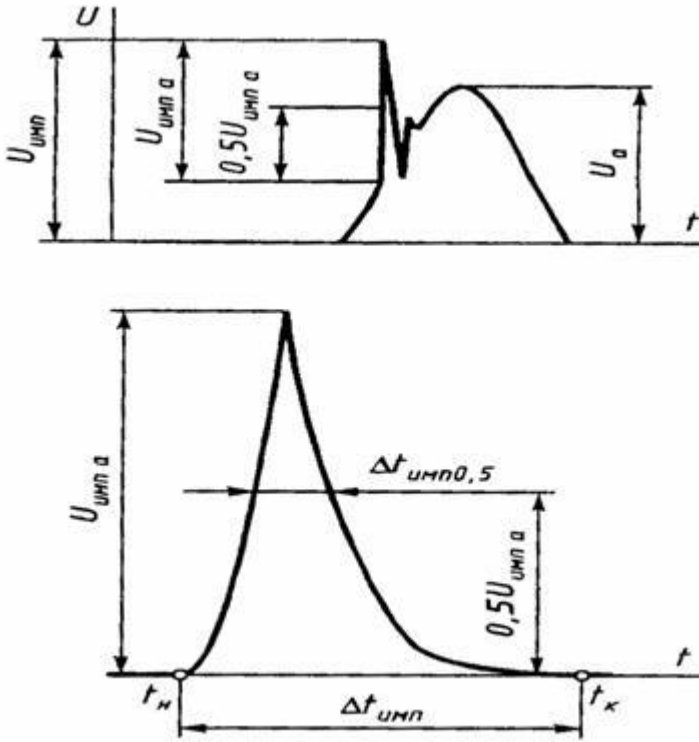
Рисунок Б.3 - Параметры импульсного напряжения
