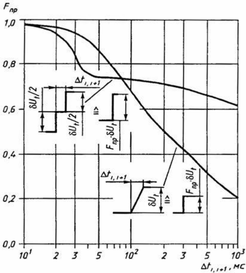
Рисунок В.1 - Коэффициент приведения F_{np} для периодических колебаний напряжения, имеющих двухступенчатую и пилообразную форму
