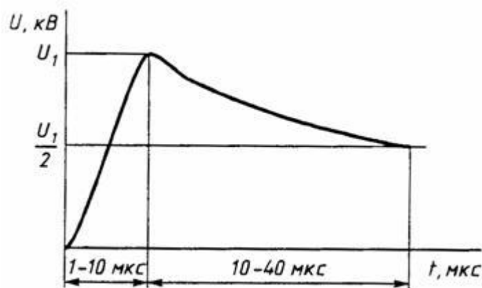
Рисунок Д.4 - Форма грозových импульсов, характерная для точек присоединения б, е, ж на рисунке Д.1.
