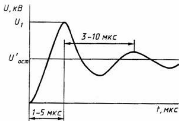
Рисунок Д.3 - Форма грозových импульсов, характерная для точек присоединения, проходящих через выводы силового трансформатора, рассматриваемая обмотка которого имеет связь с ВЛ (точки присоединения з, зϕ, и на рисунке Д.1)
