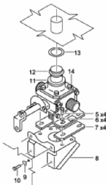
Рисунок А.1 - Пример указания количества одинаковых деталей
