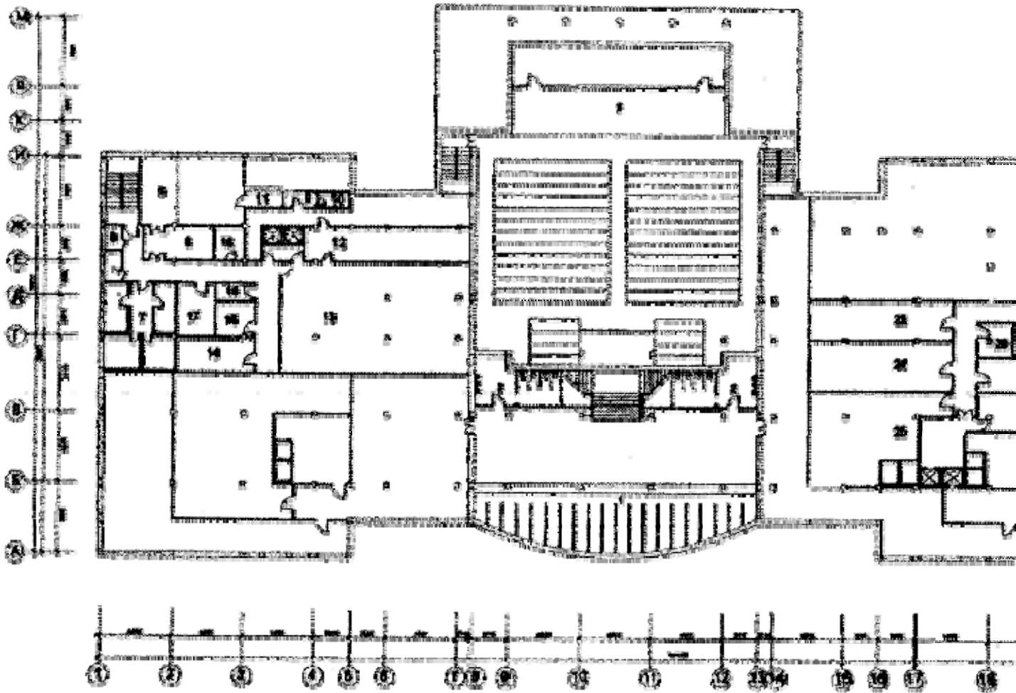
Рисунок Я.2 - План цокольного этажа
