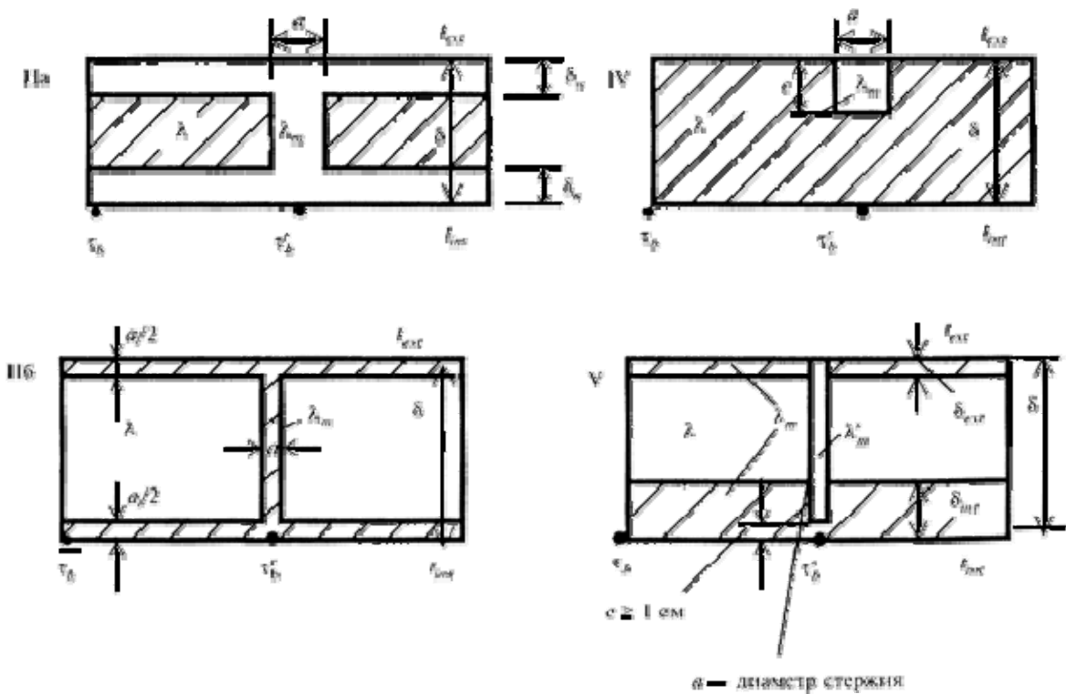
Рисунок Н.1 - Схемы теплопроводных включений в ограждающих конструкциях
