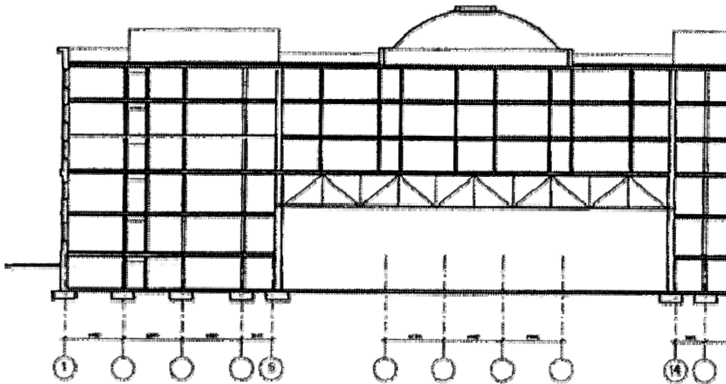
Рисунок Я.3 - Продольный разрез
