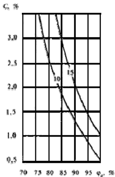
Рисунок Щ.6 - Изолинии сорбционного влагосодержания керамзитобетона \rho_0 = 1200 \text{ кг/м}^3 , содержащего NaCl - 30%, KCl - 60%, \text{MgCl}_2 - 10%, при изменении относительной влажности воздуха \varphi_a , %, и массового солесодержания C , %, в стенах цехов сушки
