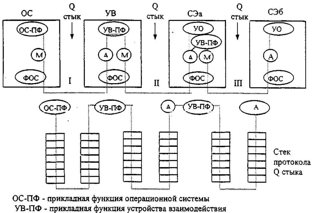
Рисунок 3 - Примеры организации связи при управлении сетью
