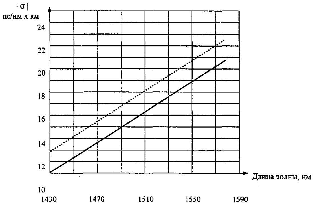
Рисунок А.3 - Максимальная абсолютная величина коэффициента дисперсии |\sigma| для ОК по [24] (—) и по [25] (-----) в диапазоне длин волн 1550 нм
