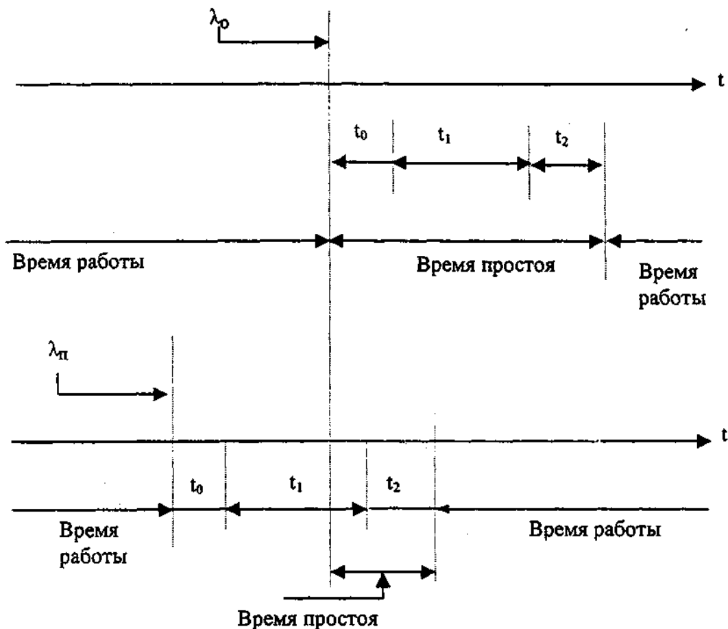
Рисунок 7 - Схема функционирования ОТЭ
