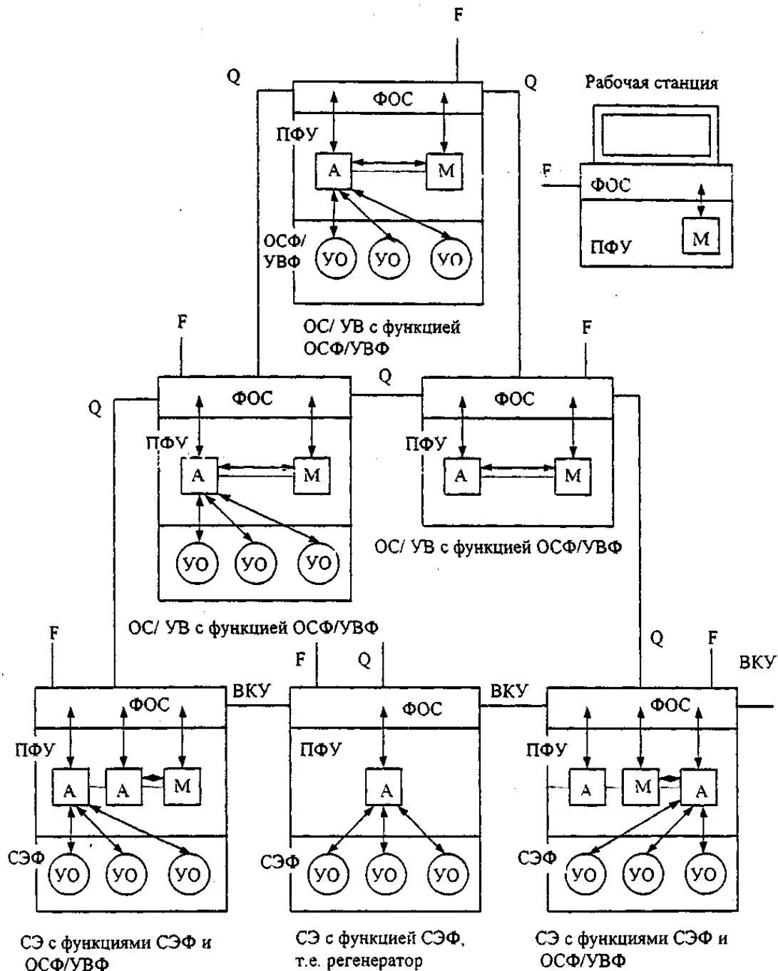
Рисунок 2 - Модель организации управления сетью ЦСП СЦИ
