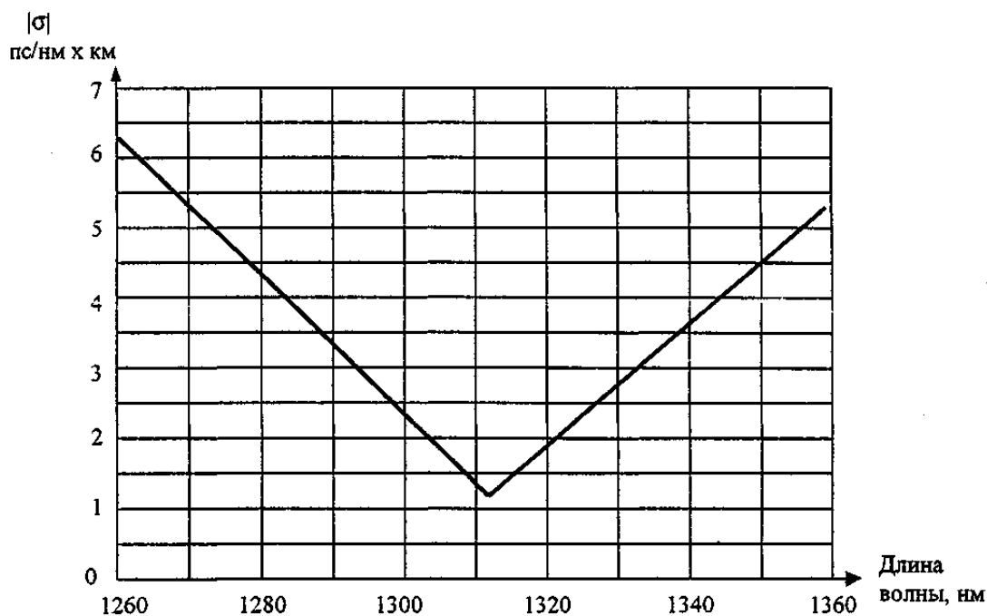
Рисунок А. 2 - Максимальная абсолютная величина коэффициента дисперсии |\sigma| для ОК по [24] в диапазоне длин волн 1310 нм
