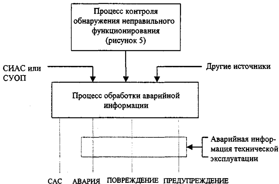
Рисунок 6 - Процесс обработки аварийной информации
