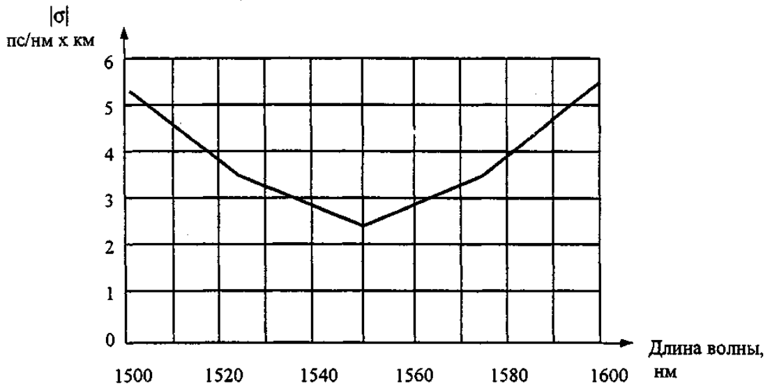
Рисунок А.4 - Максимальная абсолютная величина коэффициента дисперсии |\sigma| для ОК по [25]
