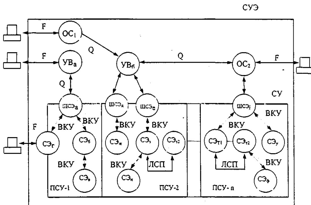
Рисунок 4 - Модель СУ, ПСУ и СУЭ
