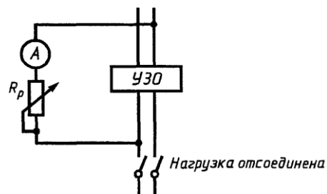
Рисунок В.2 — Схема проверки УЗО по методу 2
