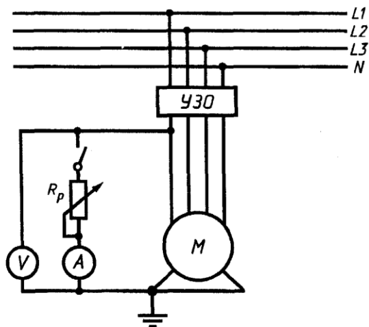
Рисунок В.1 — Схема проверки УЗО по методу 1
