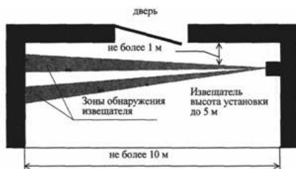
Вариант 4. Блокировка двери на проникновение извещателями магнитоконтактным и поверхностным оптико-электронным с зоной обнаружения типа "занавес"
