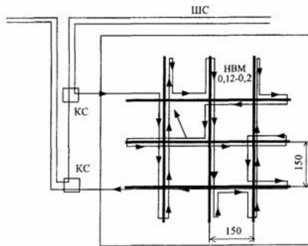
Вариант 2. Блокировка неоткрывающихся решеток проводом
