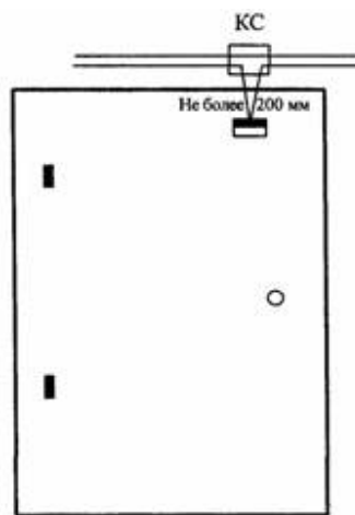
Вариант 2. Блокировка двери на открывание извещателем магнитоконтактным
