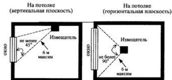
Вариант 5. Блокировка окна на открывание и разбитие извещателем магнитоконтактным и поверхностным звуковым
