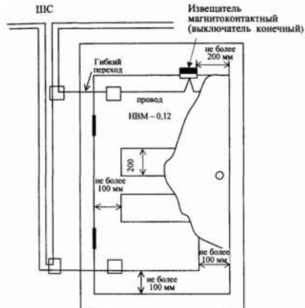
Вариант 1. Блокировка дверей (калиток) на открывание - извещателем магнитоконтактным, на разрушение - проводом
