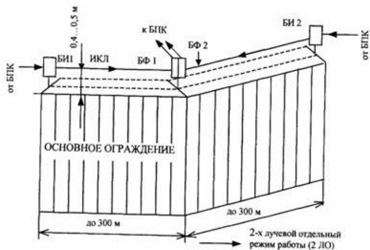
Вариант 3. Блокировка основного ограждения извещателем активным оптико-электронным
