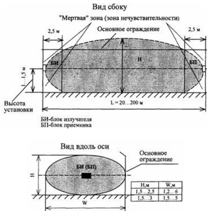
Вариант 4. Блокировка основного ограждения извещателем линейным радиоволновым
