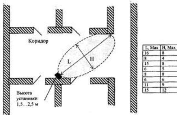
Вариант 4. Блокировка коридора извещателем объемным радиоволновым (комбинированными)
