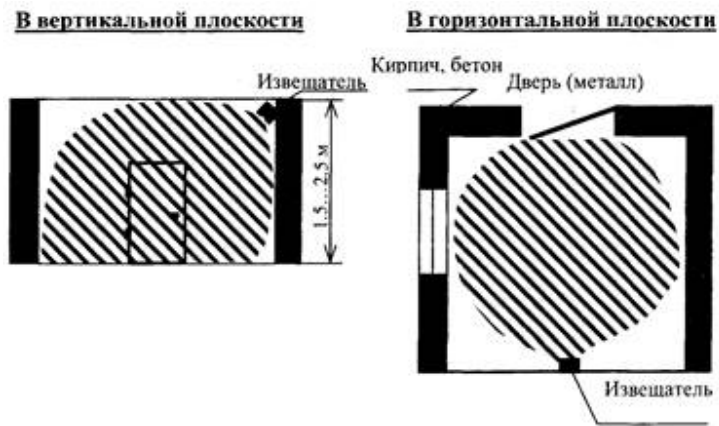
Вариант 7. Блокировка двери на открывание и проникновение извещателем объемным радиоволновым (комбинированным)
