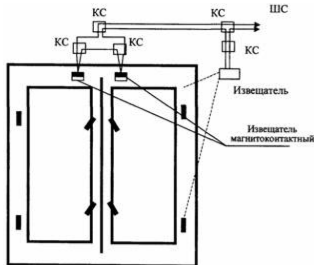
Вариант 5. Блокировка окна на открывание и разбитие извещателем магнитоконтактным и поверхностным звуковым
