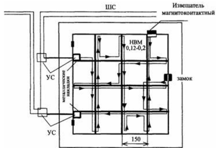
Вариант 3. Блокировка открывающихся решеток проводом
