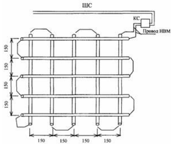
Вариант 1. Блокировка фальшрешетки проводом
