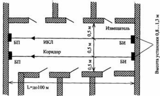
Вариант 1. Блокировка коридора извещателями активными линейными оптико-электронными
