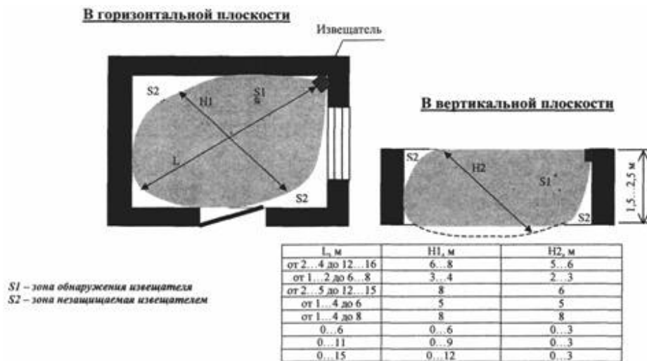
Вариант 1. Одновременная блокировка на проникновение стен, потолка, пола, а также объема помещения извещателем объемным радиоволновым (комбинированным)
