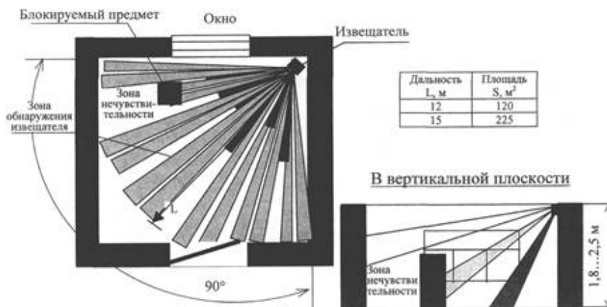
Вариант 7. Одновременная блокировка объема и отдельных предметов опико-электронным извещателем
