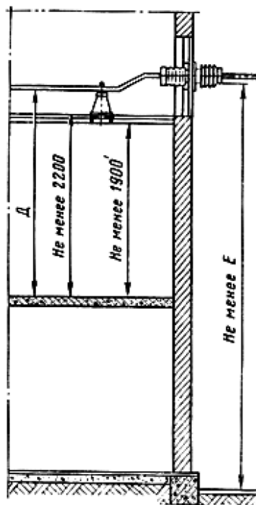
Рис. 4.2.15. Наименьшие расстояния от пола до неогражденных неизолированных токоведущих частей и до нижней кромки фарфора изолятора и высота прохода в ЗРУ.
